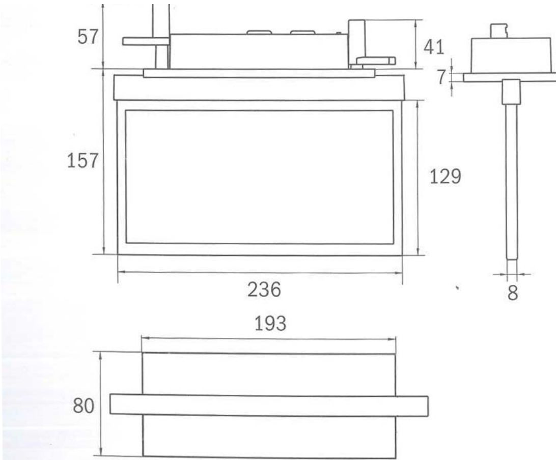
Maße AM Wandeinbaumontage
