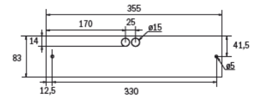
Bohrabstände Decke / Wand Drill holes ceiling / wall distances de perçage
