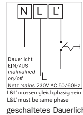
geschaltetes Dauerlicht
