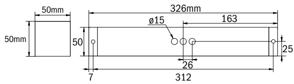
Maße und Bohrabstände KB Wand / Decke Dimensions and drilling distances KB wall / ceiling
