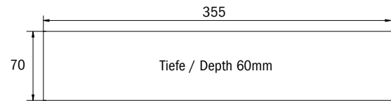
Lochausschnitt KB Einbaurahmen Hole cut-out KB recessed frame
