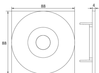
Lochausschnitt EER / EEQ
