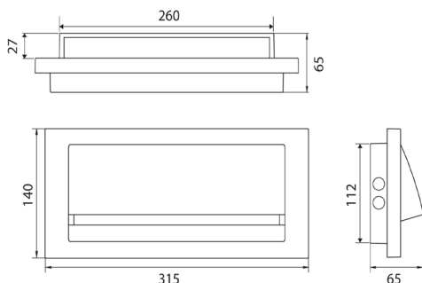
Maße Deckenaufbau
